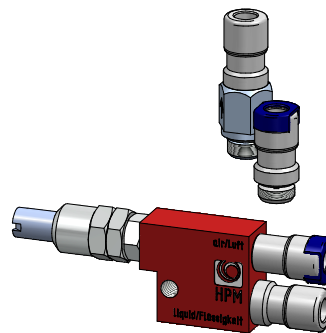
55 00 0031.001 Sprühkopfgruppe-HTRR050-05x10-AL Spray head group
